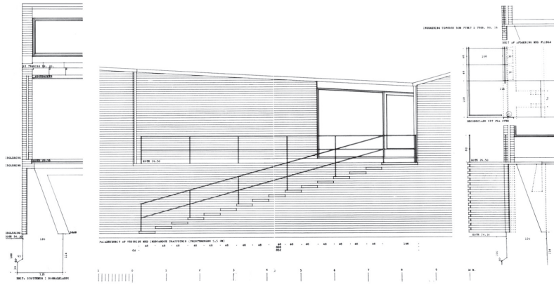
Sección transversal y alzado. Cross section and elevation.
